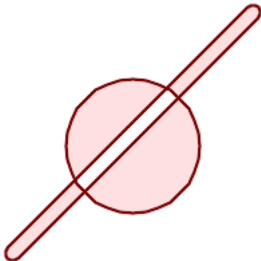
after_geom : 具有四个非重多边形形成的多边形
