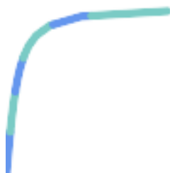
致密 \boxtimes 和分割 \boxtimes 。
