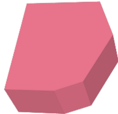
geom1 和 geom2 的交集
