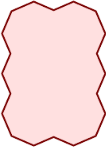
after_geom_structure : 由一个非重叠多边形组成的多边形
