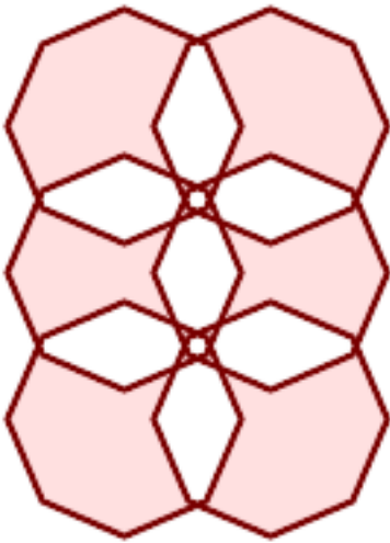
after_geom : 由 14 个不重叠多边形组成的多边形
