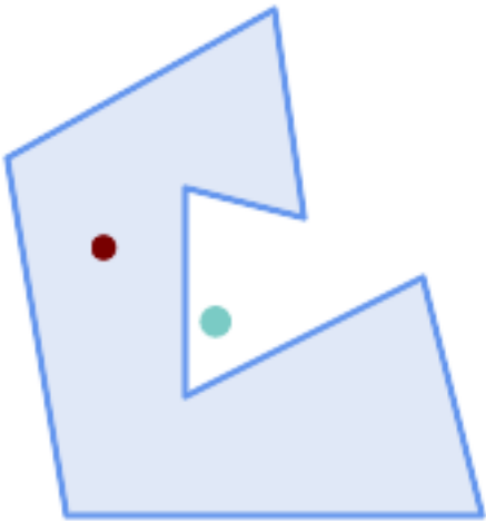
绿色：表面上的点；红色：重心
